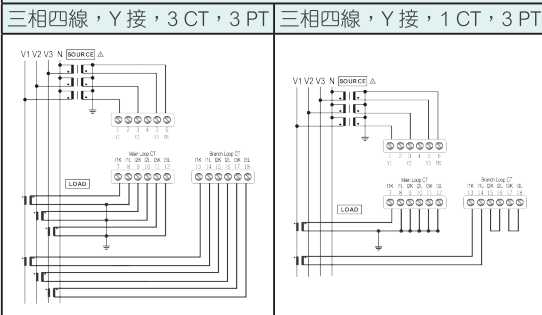
主迴路 CT 二次側為 333mV 訊號
