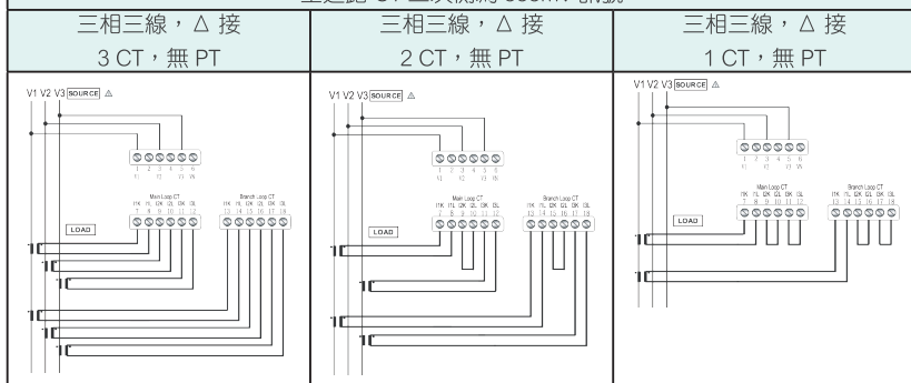
主迴路 CT 二次側為 333mV 訊號
